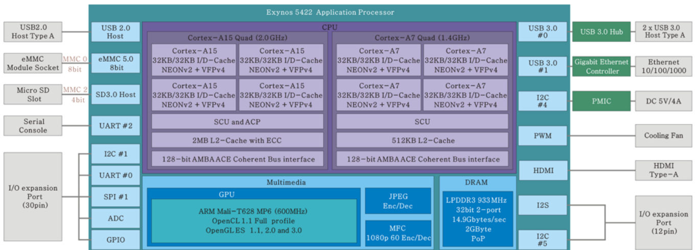
ODROID-XU4 BLOCK DIAGRAM
